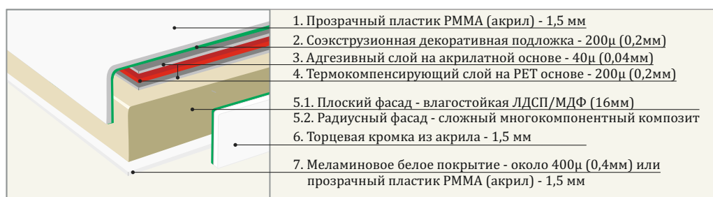
Коллекция Brilliantlinie. Структура фасада.
