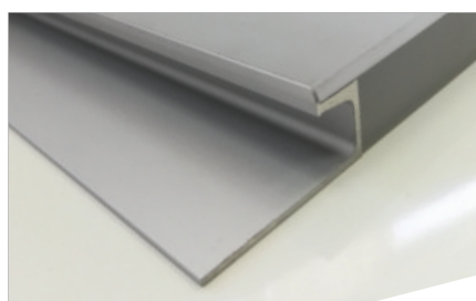
Нижний фасад с верхней интегрированной ручкой артикул ИР-1.
