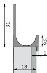
Нижний фасад с верхней интегрированной ручкой артикул ИР-3.
