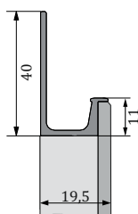
Нижний фасад с верхней интегрированной ручкой артикул ИР-1.
