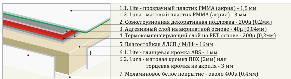
Коллекция Lite/Luna. Структура фасада.
