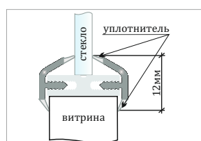
схематическое изображение декоративного профиля
